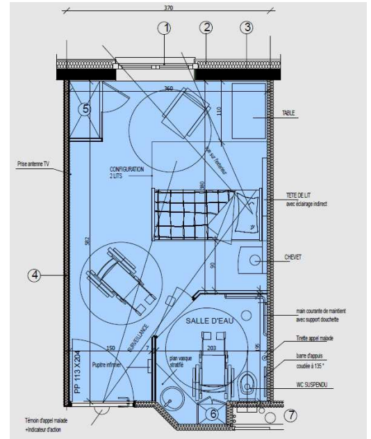
Plan de chambre type
